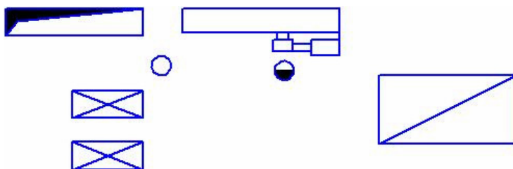
Рис. 2.10. Организация рабочего места вертикального форматно-раскrojного станка модели COMPACT 4164 фирмы « STRIEBIG » (Швейцария) для раскrojа древесно-стружечных плит ПСП, ОСВ, фанеры, гипсокартона, массива древесины
