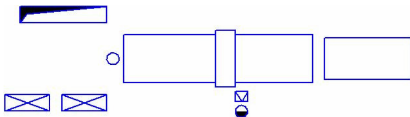
Рис. 2.10. Организация рабочего места вертикального форматно-раскrojного станка модели COMPACT 4164 фирмы « STRIEBIG » (Швейцария) для раскrojа древесно-стружечных плит ПСП, ОСВ, фанеры, гипсокартона, массива древесины
