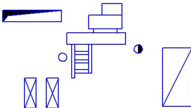
Рис. 2.9. Организация рабочего места форматно-раскrojного станка модели WT-3000 фирмы « ATLENDORF » (Германия)
