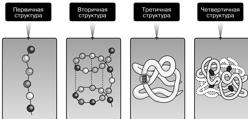
Рис. 10. Структуры белка
