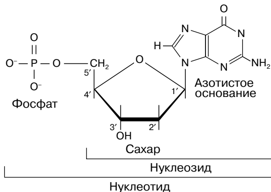
Рис. 11. Нуклеотид
