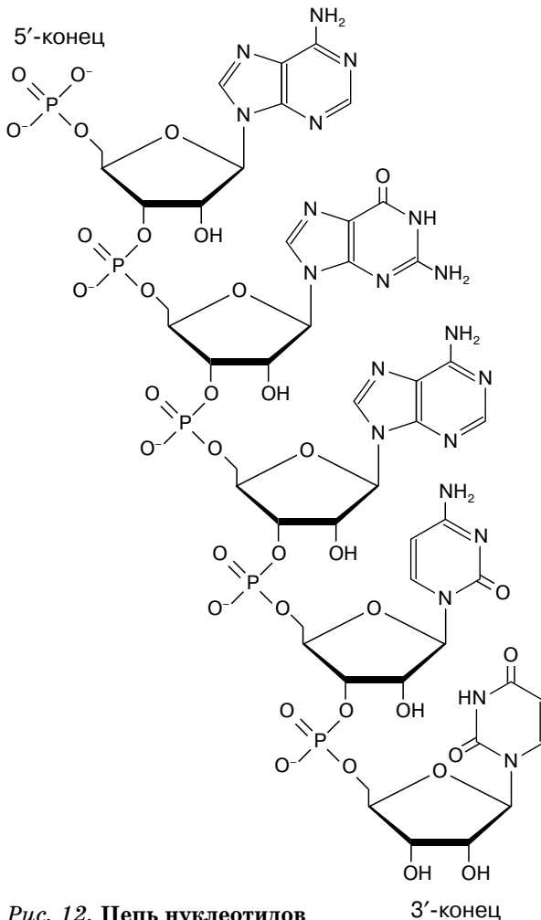
Рис. 12. Цепь нуклеотидов
