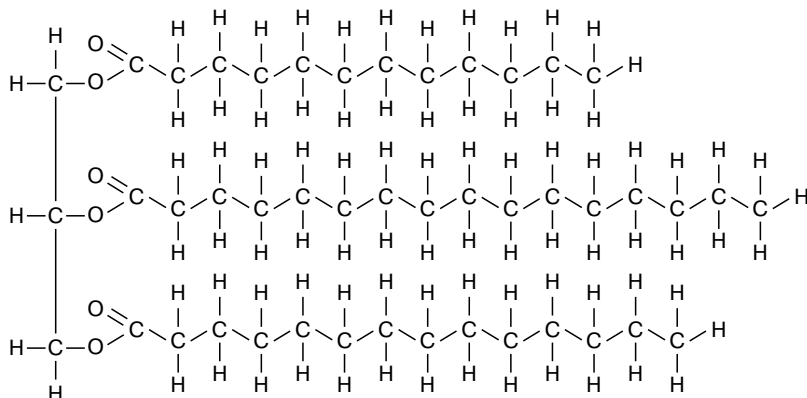
Рис. 7. Молекула жира
