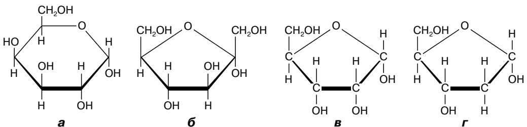
Рис. 4. Моносахариды:
