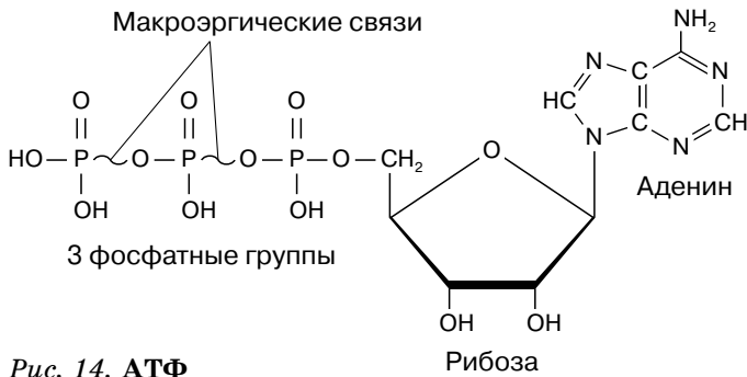
Рис. 14. АТФ
