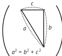
Рис. 4 Теорема Пифагора
