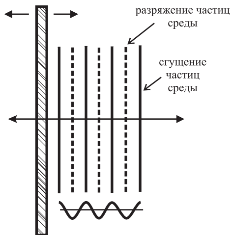
Рис. 1.1. Плоская волна
