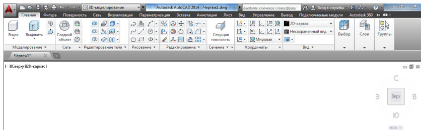
Рис. 1.7. Пространство 3D-моделирование
