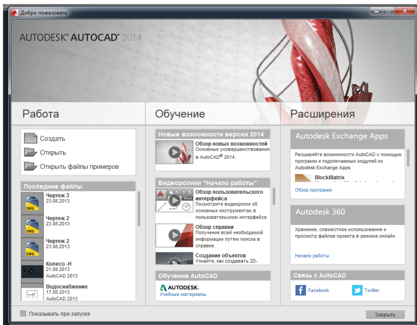
Рис. 1.1. Окно приветствия
