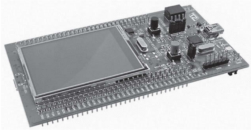
Рис. 1.3. Внешний вид отладочной платы «STM32F469I-DISCO» [1-8]
