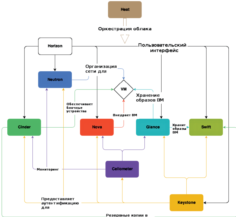
Рис. 1.2. Архитектура OpenStack
