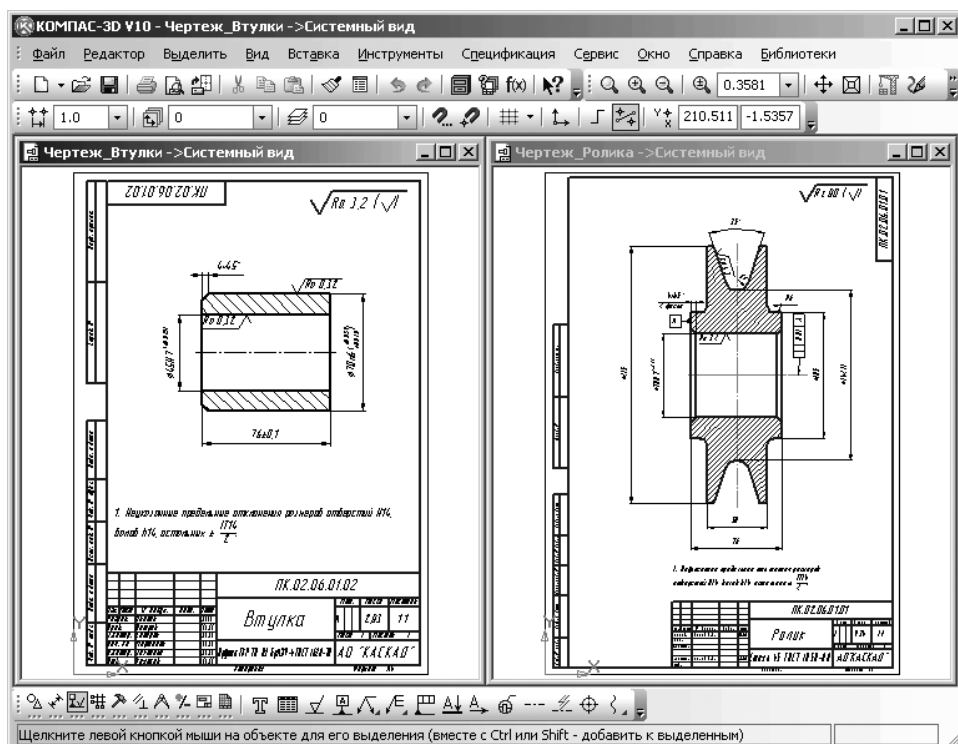
Рис. 6.1. Представление деталей перед созданием сборочного чертежа Ролик_Втулка
