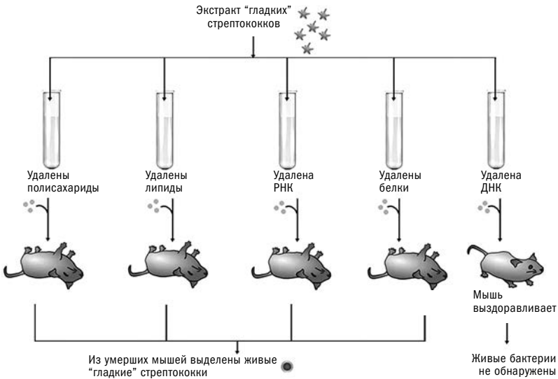
Рис. 3. Опыт Эвери – Маклеода – Маккарти
