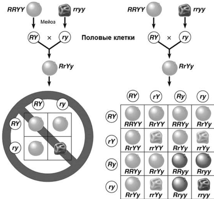
Рис. 1. Так работает закон независимого распределения признаков, открытый Менделем. Пусть “наследственный задаток”, отвечающий за желтый цвет горошины, — Y, за зеленый — y, за гладкую горошину — R, морщинистую — r. Заглавными буквами показано доминирование, то есть преобладание признака над альтернативным: если хотя бы одна из двух R заглавная, горошина будет гладкой. В первом поколении все горошины одинаковые, а что будет во втором? Если бы признаки “желтая и гладкая”, “зеленая и морщинистая” всегда передавались вместе, мы наблюдали бы такое распределение, как показано слева. На самом деле признаки комбинируются в различных сочетаниях — появляются растения с желтыми морщинистыми и зелеными гладкими горошинами. Значит, наследственные задатки, отвечающие за цвет и за форму, независимы друг от друга!
