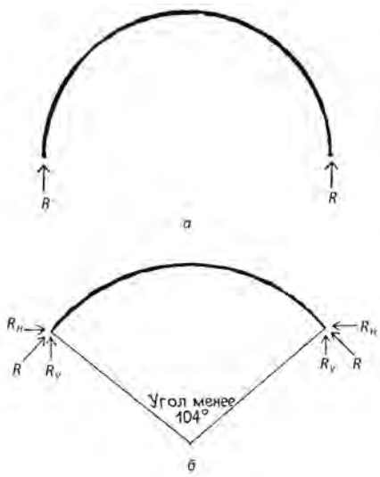
Рис. 1.1. Реакция в полусферическом куполе и плоском куполе
