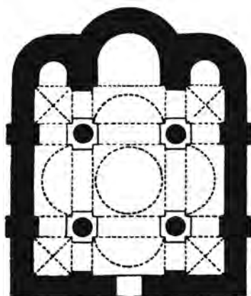
Рис. 1.13. Церковь св. Иоанна Предтечи. План (Керчь, Крым)
