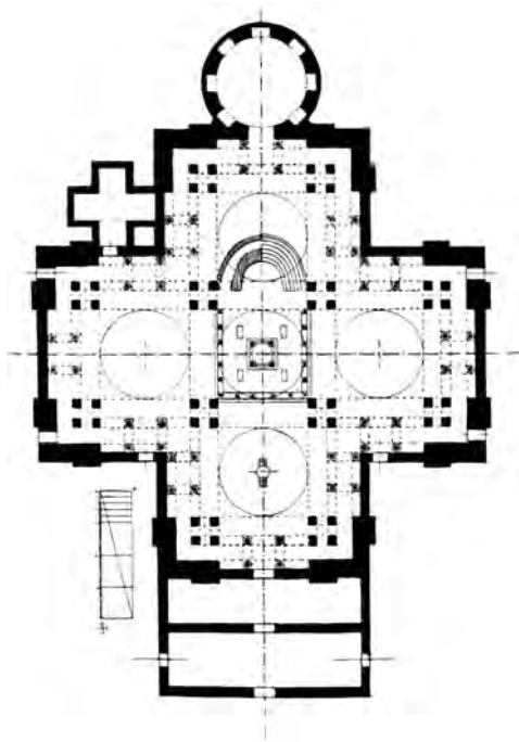
Рис. 1.5. Церковь св. Апостолов в Константинополе. План (реконструкция) (Стамбул, Турция)
