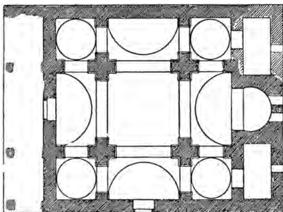
Рис. 1.12. Церковь вне стен Русафы. План (Сирия)
