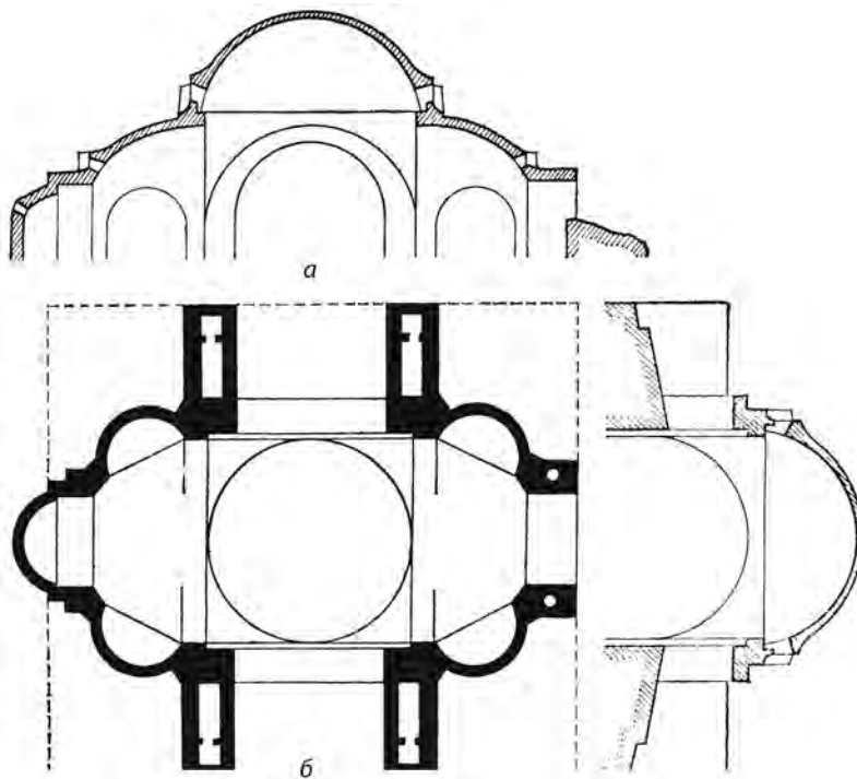
Рис. 1.3. Собор св. Софии в Константинополе (Стамбул, Турция): а — разрез; б — план
