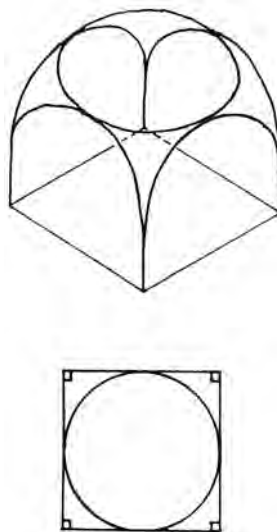
Рис. 1.2. Превращение циркульного плана плоского сферического купола в квадрат
