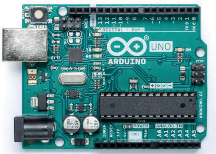
Рис. 1 ❖ Лицевая сторона оригинальной платы Arduino Uno
