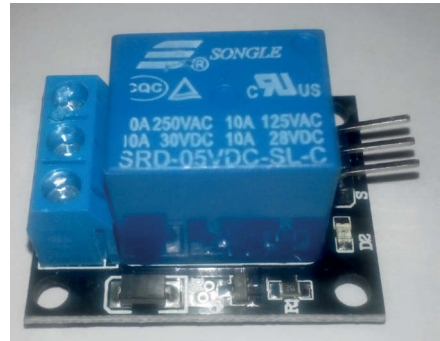
Рис. 22 ❖ Релейный модуль
