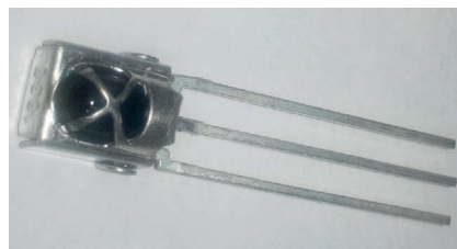
Рис. 28 ❖ Инфракрасный приемник управления NEC
