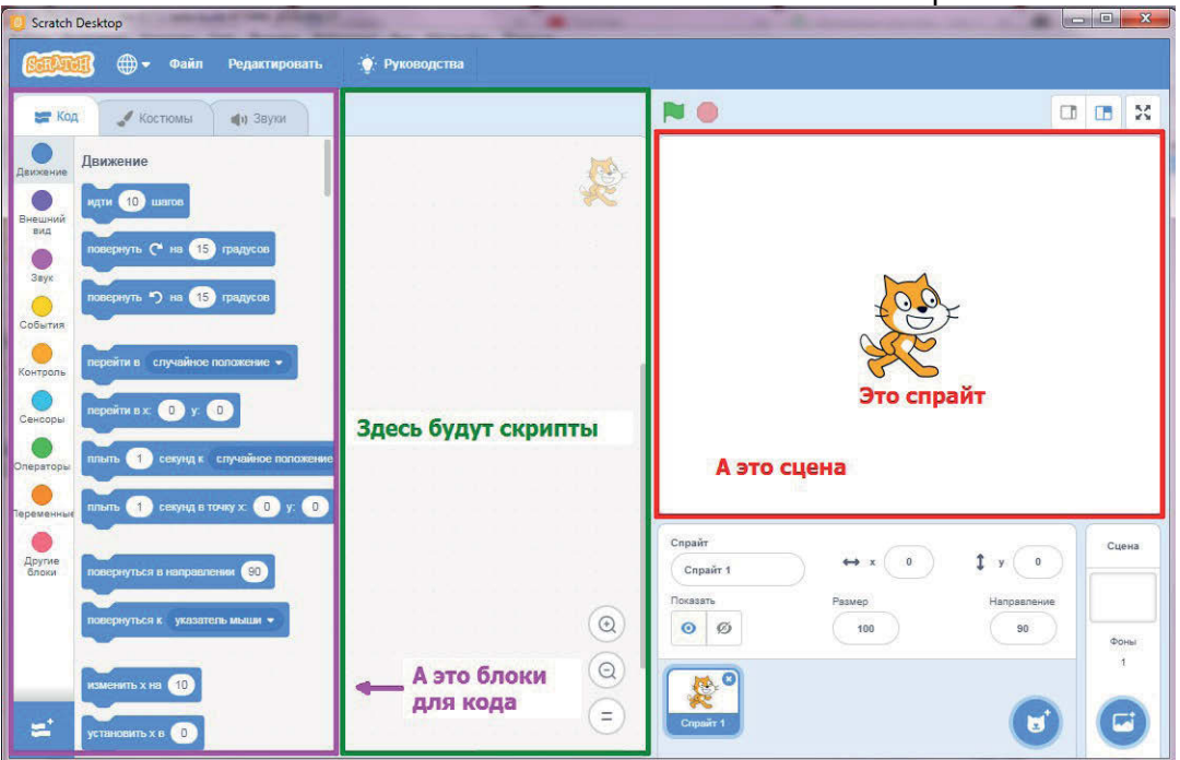
Рис. 5. Структура Scratch
