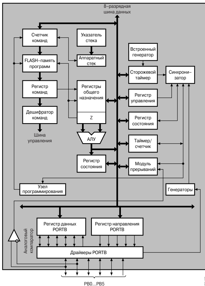
Рис. 1.6. Структурная схема микроконтроллеров ATtiny11/11L
