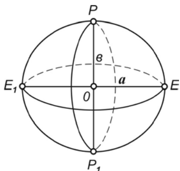
Рис. 1. Земной эллипсоид
