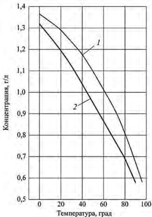
Рис. 14. Растворимость \text{Ca}(\text{OH})_2 и \text{CaO} в зависимости от температуры: 1 — \text{CaO} ; 2 — \text{Ca}(\text{OH})_2
