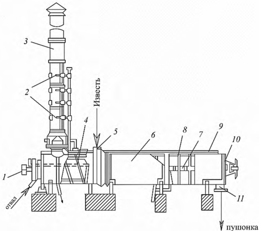
Рис. 12. Гидратор непрерывного действия для гашения в пушонку:
