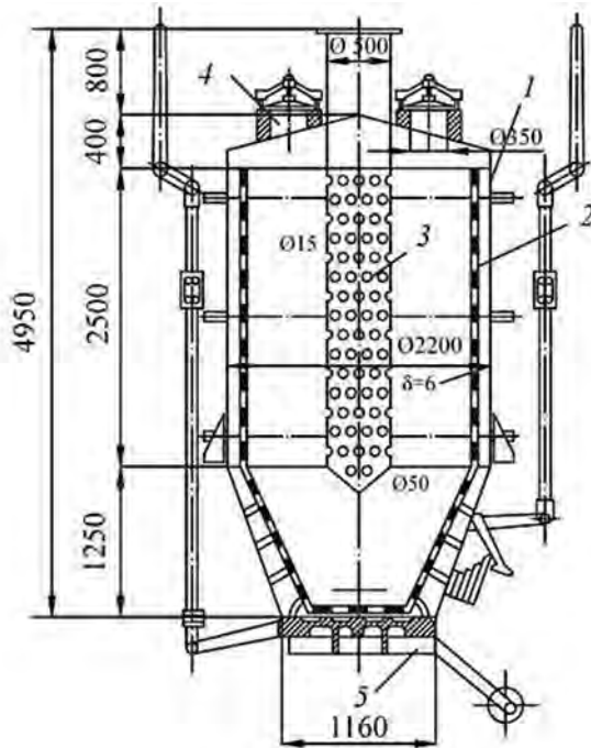
Рис. 4. Запарочный аппарат:
