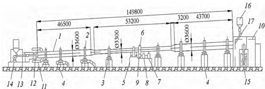
Рис. 15. Вращающаяся печь длиной 150 м:
