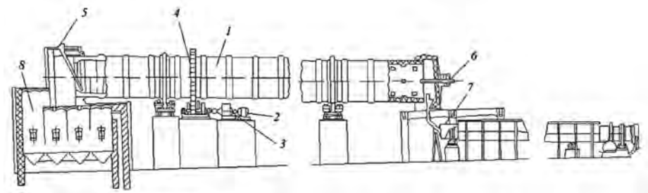
Рис. 10. Вращающаяся печь для обжига извести:
