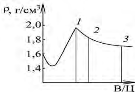
Рис. 16. График зависимости средней плотности цементного теста от водоцементного отношения ( V/C ):
