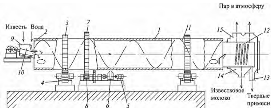
Рис. 13. Гаситель барабанного типа для гашения извести в молоко:
