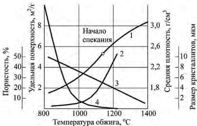
Рис. 8. Зависимость средней плотности, пористости, внутренней удельной поверхности и размера кристаллов извести от температуры обжига \text{CaCO}_3 : 1 — средняя плотность; 2 — размер кристаллов; 3 — пористость; 4 — удельная поверхность
