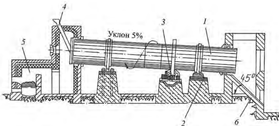
Рис. 3. Схема производства строительного гипса с обжигом во вращающихся печах (сушильных барабанах):
