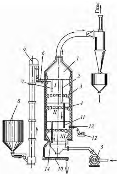
Рис. 11. Схема установки для обжига извести в кипящем слое:
