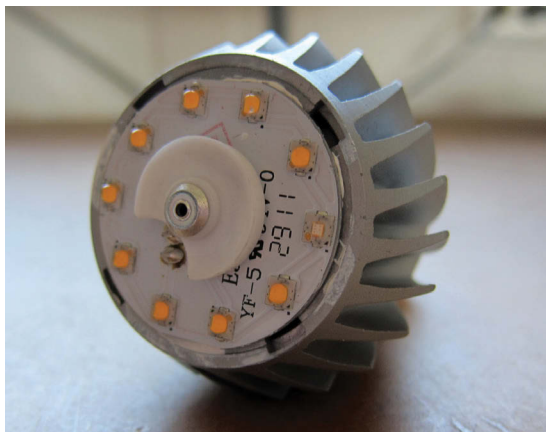
Рис. 1.10. Внешний вид разобранной светодиодной лампы
