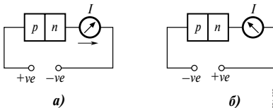
Рис. 1.9. p-n-переход в качестве выпрямителя: а — прямое смещение; б — обратное смещение.
