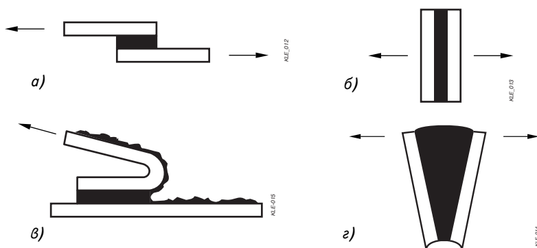
Рис. 4. Основные типы напряжений: а — сдвиг; б — равномерный отрыв или симметричное растяжение; в — отдира; г — внецентренное растяжение
