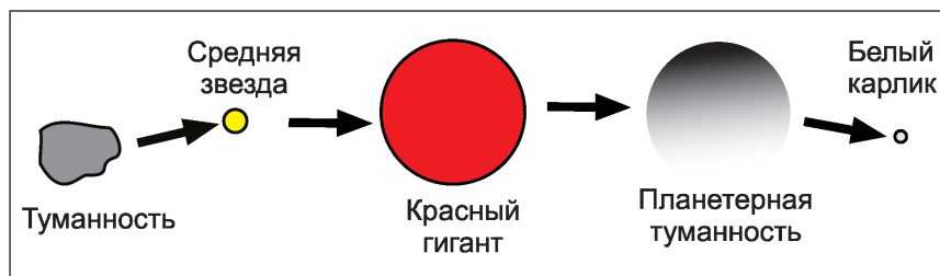
Рис. 9. Жизненный цикл звезды
