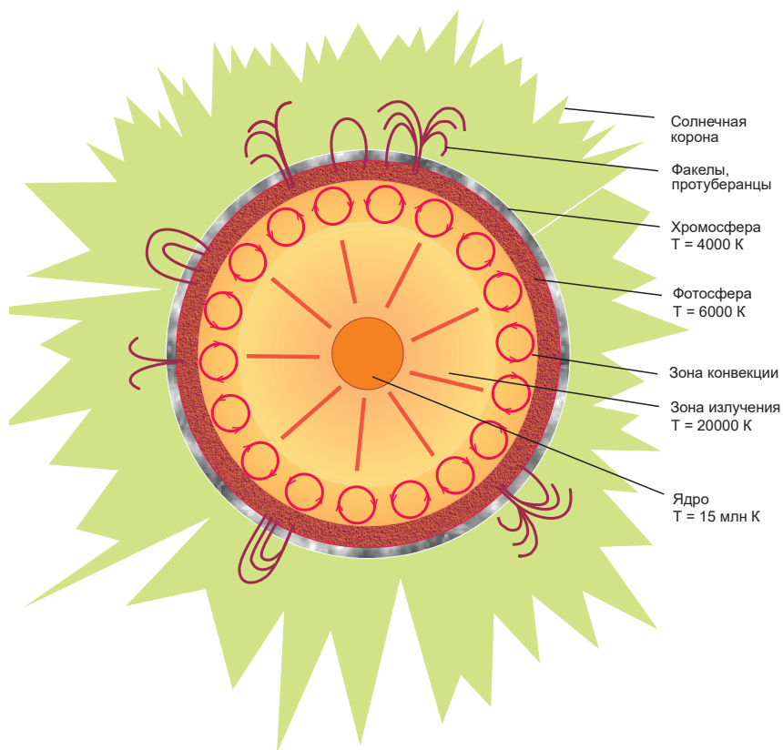
Рис. 6. Строение Солнца (из кн.: Короновский, Брянцева, 2019)
