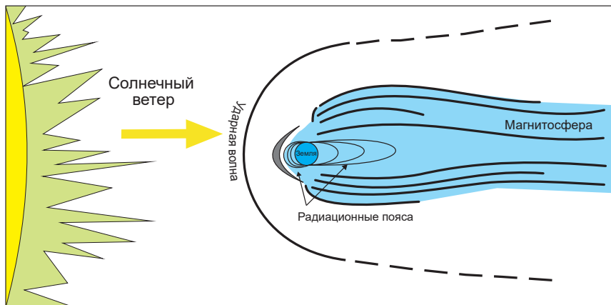
Рис. 7. Действие солнечного ветра – потока плазмы – на магнитосферу Земли (из кн.: Короновский, Брянцева, 2019; упрощенно)
