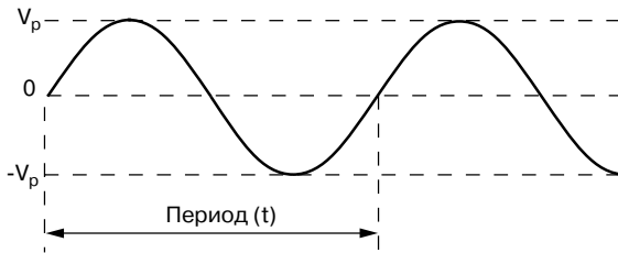
Рис. 1.1. Синусоидальная волна
